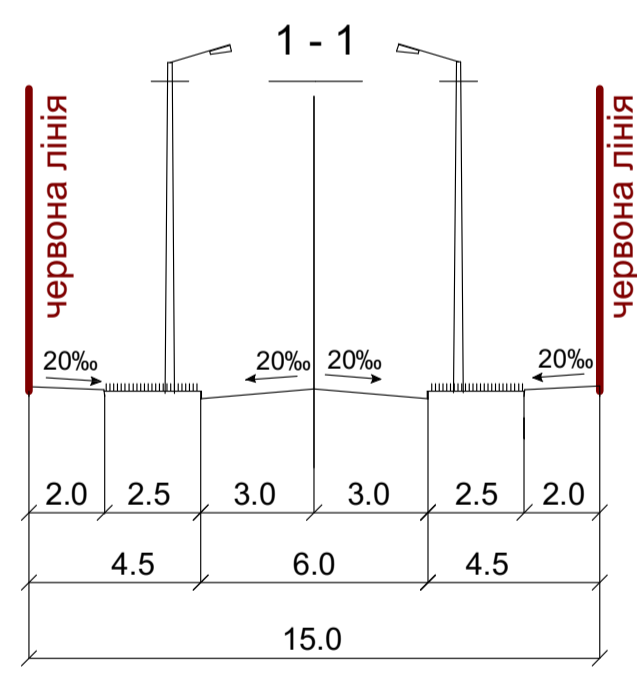
Поперечний профіль
