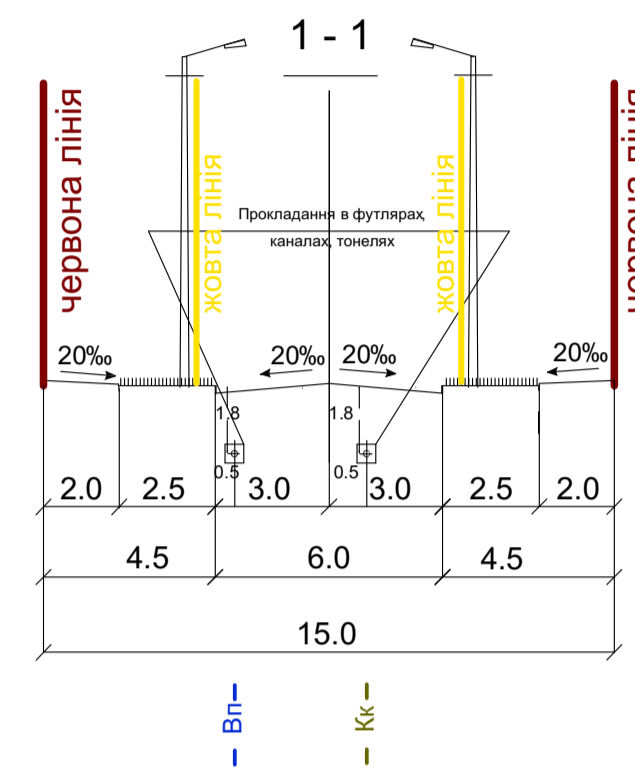
Поперечний профіль
